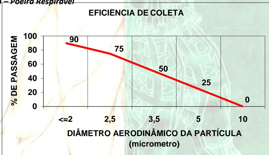
Gráfico 4 – Poeira Respirável
